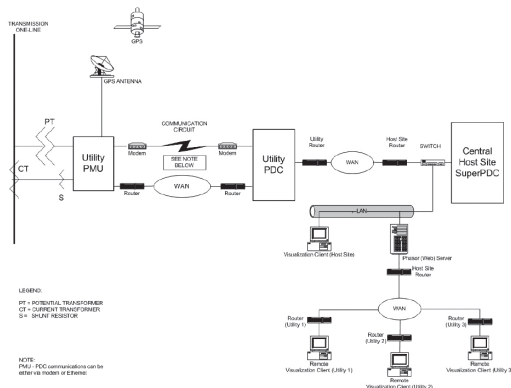
Figura 3: Sistema de comunicaciones típica de un PMU
