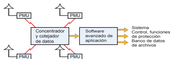
Figura 4: Típica red fasorial
