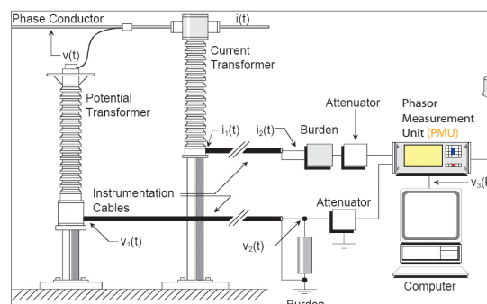
Figura 5: Implementación típica de un PMU en una subestación
